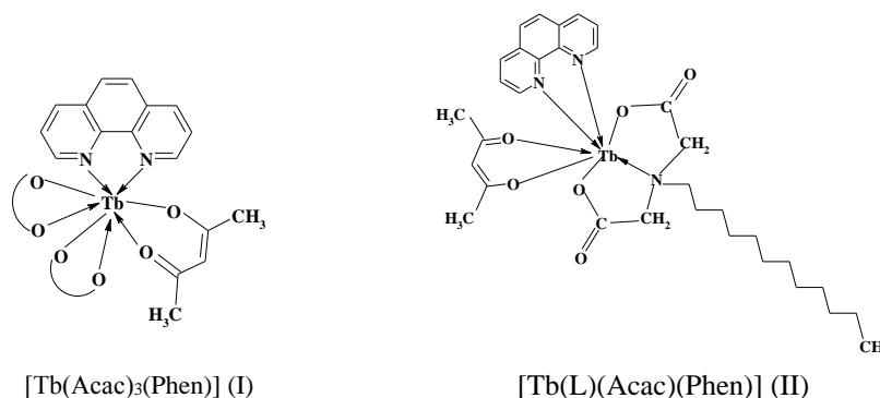
Рис. 1. Структура синтезированных координационных соединений тербия(III)
