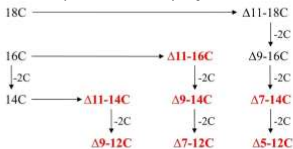
Рис. 3. Возможные пути биосинтеза компонентов половых феромонов Lepidoptera . Красным цветом выделены варианты длинноцепочечных углеводородных радикалов аттрактивных молекул Zygaenidae
