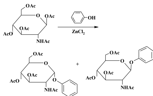
Рис. 1. Общая схема синтеза фенол-2-ацетида-3,4,6-три-О-ацетил-2-дезоксi-α-D-глюкопиранозида и его аномера в условиях сплавления с ZnCl_2
