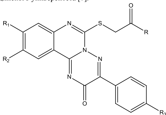
Рисунок 1 - Общая формула исследуемых производных NKV, где R – OH, C n H m O x F y N z Br q ; R 1 – F, Cl, Br, I, H, O–CH 3 , C 6 H 5 ; R 2 , R 3 – F, Cl, Br, I, H.
