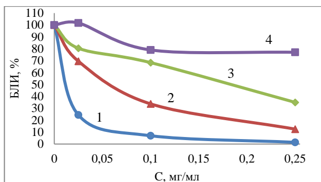
Рисунок 3 - Влияние ЛП и производных NKV на биолюминесценцию тест-штамма P. leiognathi Sh1, где, 1 - сильные ингибиторы, 2 - ингибиторы, 3 - умеренные ингибиторы, 4 - нейтральные вещества.
