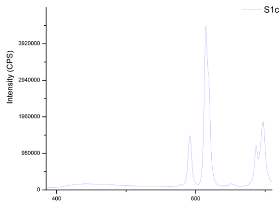
Рис. 2. Спектр люминесценции твёрдого образца комплекса [Eu(L)(Acac)(Phen)].
