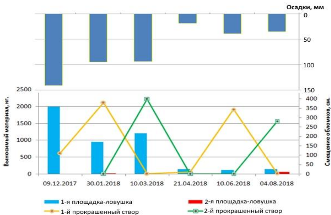
Рис. 1. Динамика развития склоновых (ломаные) и русловых (нижние столбики) процессов в балке Флишевая в зависимости от количества осадков (верхние столбики)
