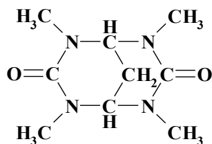
Рис. 1. Лиганд (L).
