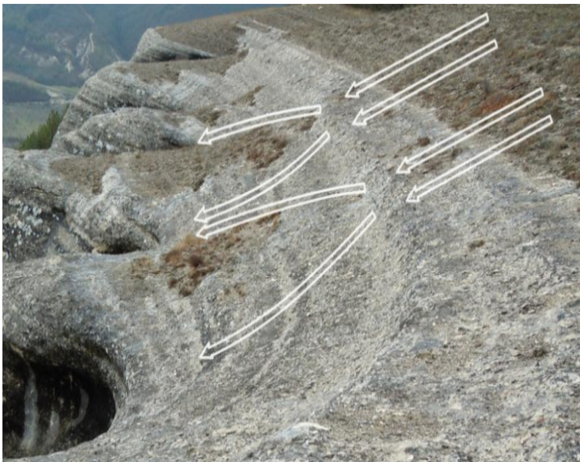
Рис. 1. Перераспределение поверхностного стока на склоне при формировании водосборных ложбин
