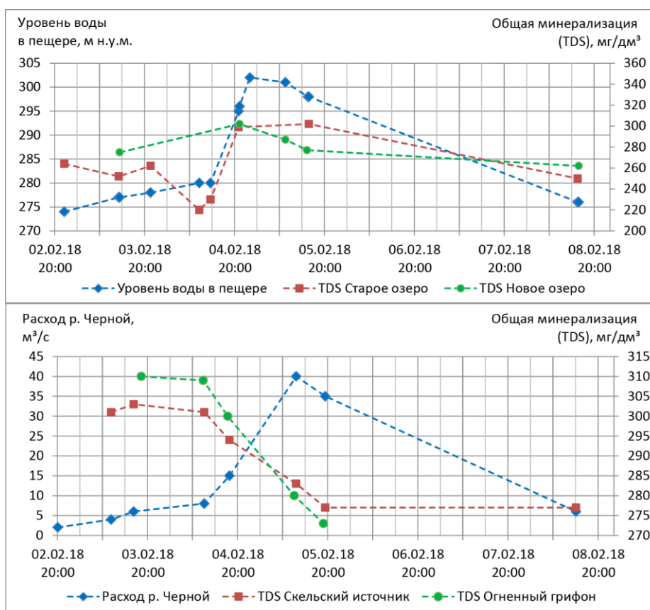
Рис. 1. Динамика гидрологических параметров в пещере Скельской и на источниках р. Черной во время паводка 02-08.02.2018.
