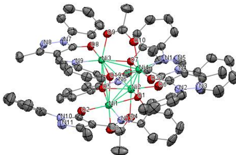
Рисунок 1. Структура комплексного аниона [\text{Ni}_4(\text{L1})_4(\text{AcO})_2]^{2-} .
