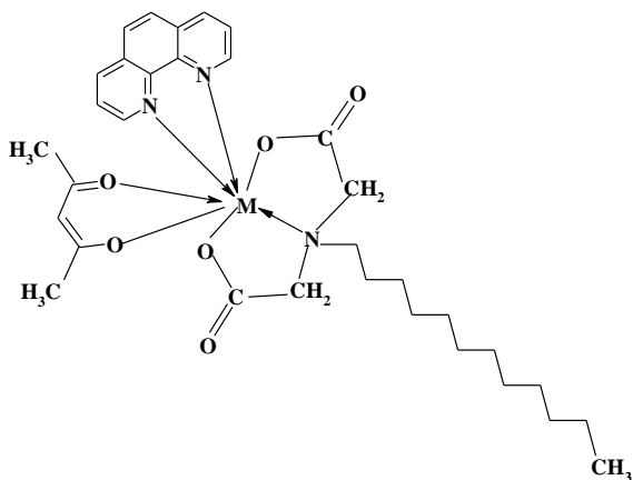
Рис. 1. Структура смешаннолигандного комплекса [Eu(L)(Acac)(Phen)].
