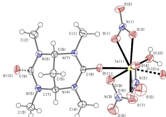
Рис. 2. Атомно-молекулярная структура I, неводородные атомы показаны на уровне 50% вероятности.
