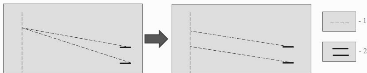
Рис.1. Изменение продольного профиля реки в зависимости от положения базиса эрозии.
