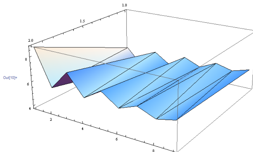
Рис.1.1. 3D решение системы (1.11) в пакете WolframMathematica 9.0.
